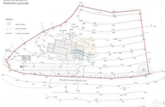
STATO DI PROGETTO Piantina generale
