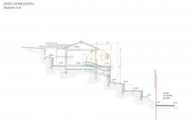
STATO DI PROGETTO Sezione X-X'
