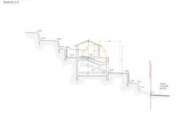
STATO DI PROGETTO Sezione Z-Z
